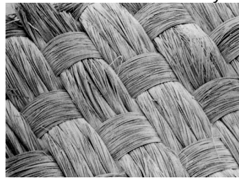
Obr. 4 Geotextilie tkaná z multivláken
