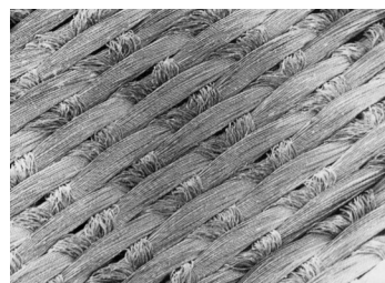
Obr. 2 Pletená geotextilie – horní povrch
