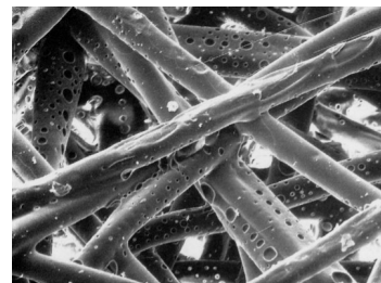
Obr. 2 Tepelně pojená netkaná geotextilie
