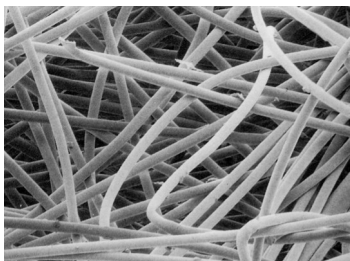
Obr. 1 Mechanicky pojená netkaná geotextilie
